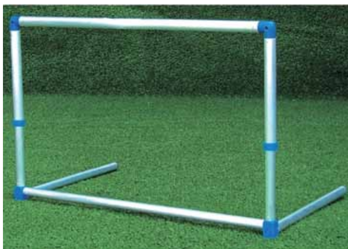
art. 3015 Ostacolo in alluminio, regolabile da 40 a 60 cm, smontabile Aluminium hurdle, adjustable cm 40 / 60
