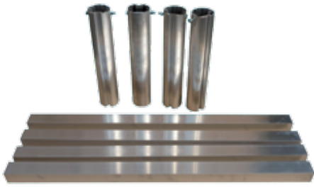
art. 6019 Kit di trasformazione da trasportabile a fissa per porte in alluminio sez. diam. 80 mm al paio Kit sochets to change freestanding soccer goal in fixed per pair
